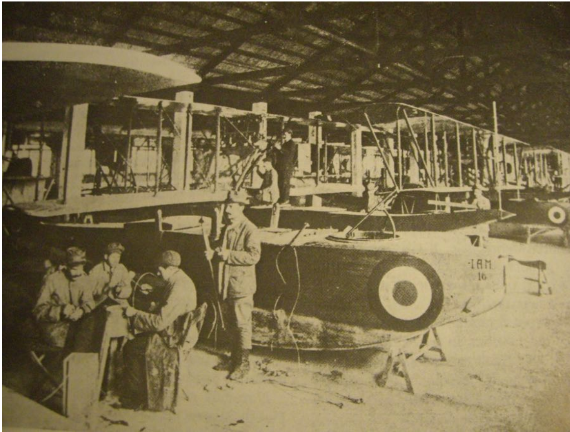
Stabilimento idrovolanti IAM Baia 1916
